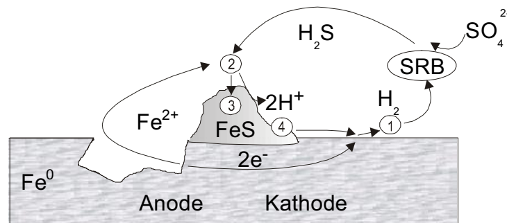
Abb. 2.2 Beteiligung von hydrogenotrophen sulfatreduzierenden Bakterien (SRB) an der anaeroben Korrosion von Stahl. Vier korrosionsfördernde Prozesse können prinzipiell ablaufen: 1. die kathodische Depolarisierung, 2. die anodische Depolarisierung (Entfernung von \text{Fe}^{2+} ), 3. die Bildung einer FeS-Schicht, die kathodisch wirken kann, 4. die Versorgung mit Protonen für die kathodische Reaktion; SRB: sulfatreduzierende Bakterien [nach CORD-RUWISCH, 2000].
