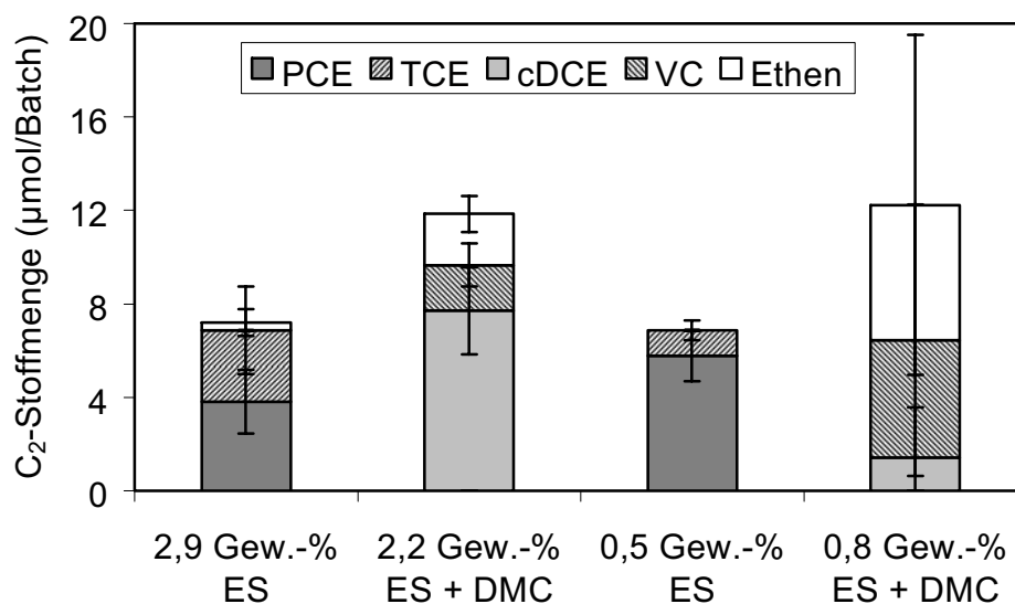
Abb. 4.24 Dechlorierung von PCE in abiotischen Ansätzen mit 2,9 und 0,5 Gew.-% ES sowie in Ansätzen mit 2,2 und 0,8 Gew.-% ES mit 2 Vol.-% DMC nach 53tägiger Inkubationszeit. Die PCE-Ausgangskonzentrationen betragen 13,1 \pm 1,1 \text{ } \mu\text{mol} .
