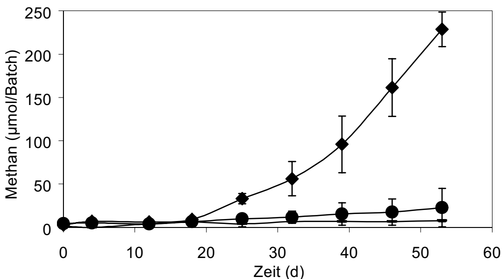
Abb. 4.25 Bildung von Methan in Ansätzen mit 2 Vol.-% DMC und 0,8 Gew.-% ES (●), bzw. 2,2 Gew.-% ES (■) sowie in Ansätzen mit H_2 (◆).
