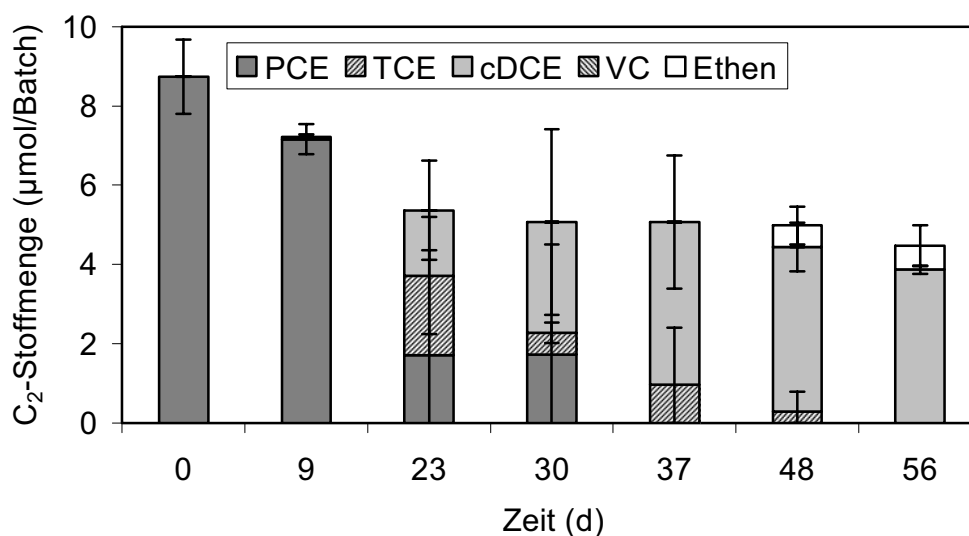
Abb. 4.11 Verlauf der PCE-Dechlorierung in Triplets mit 2 Gew.-% gealtertem GG vor der Desorption.
