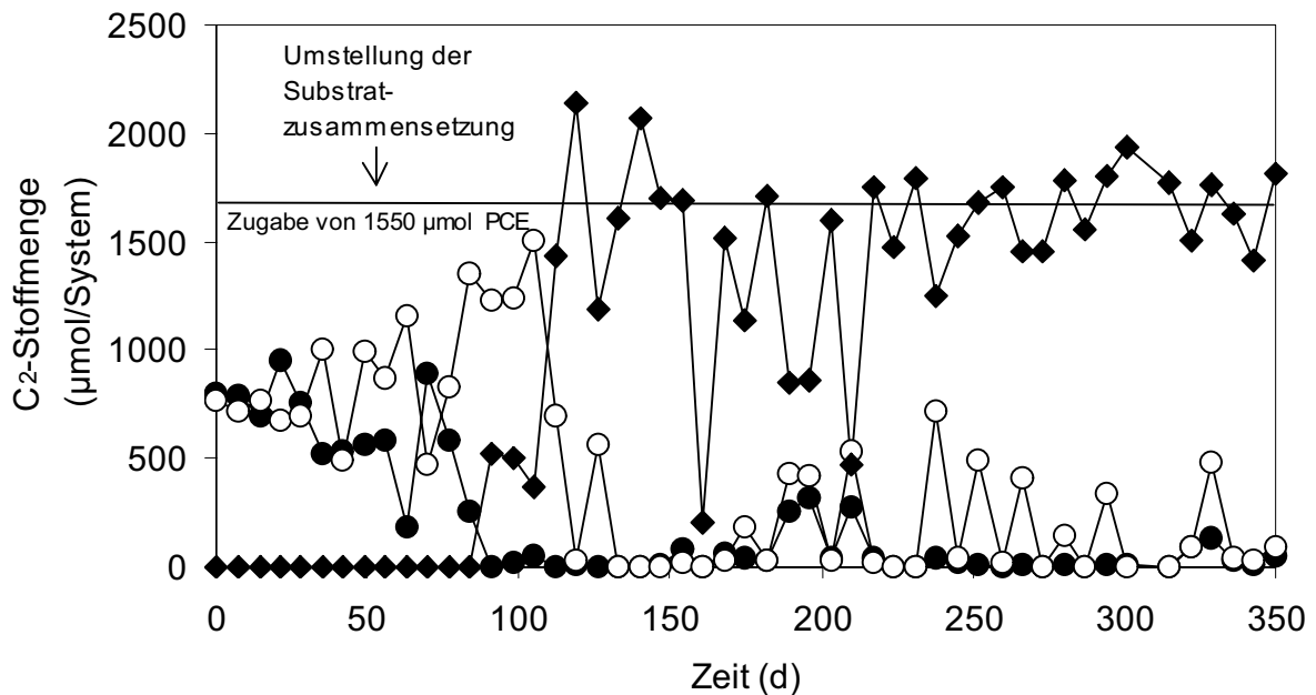
Abb. 4.15 Dechlorierung von PCE durch eine reduktiv dechlorierende Mischkultur vor und nach Substratumstellung am 51. Tag der Kultivierung. Dargestellt sind die Stoffmengen der Dechlorierungsprodukte cDCE (●), VC (○) und Ethen (◆), die jeweils eine Woche nach PCE-Zugabe gemessen wurden. PCE und TCE waren zu diesem Zeitpunkt nicht mehr nachweisbar.
