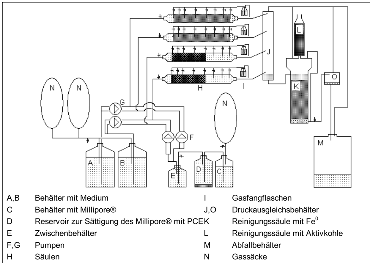
Abb. 3.2 Schema des Säulenaufbaus (BLOTEVOGEL, 2003).
