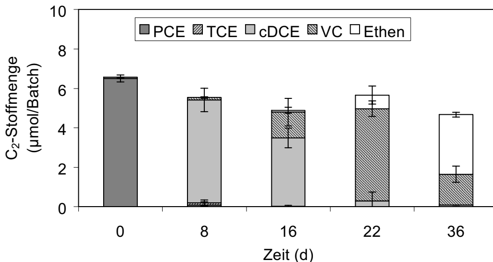
Abb. 4.27 Dechlorierung von PCE in Ansätzen mit 2 Gew.-% GG und 2 Vol.-% DMC. Die Inkubationszeit betrug 36 Tage.
