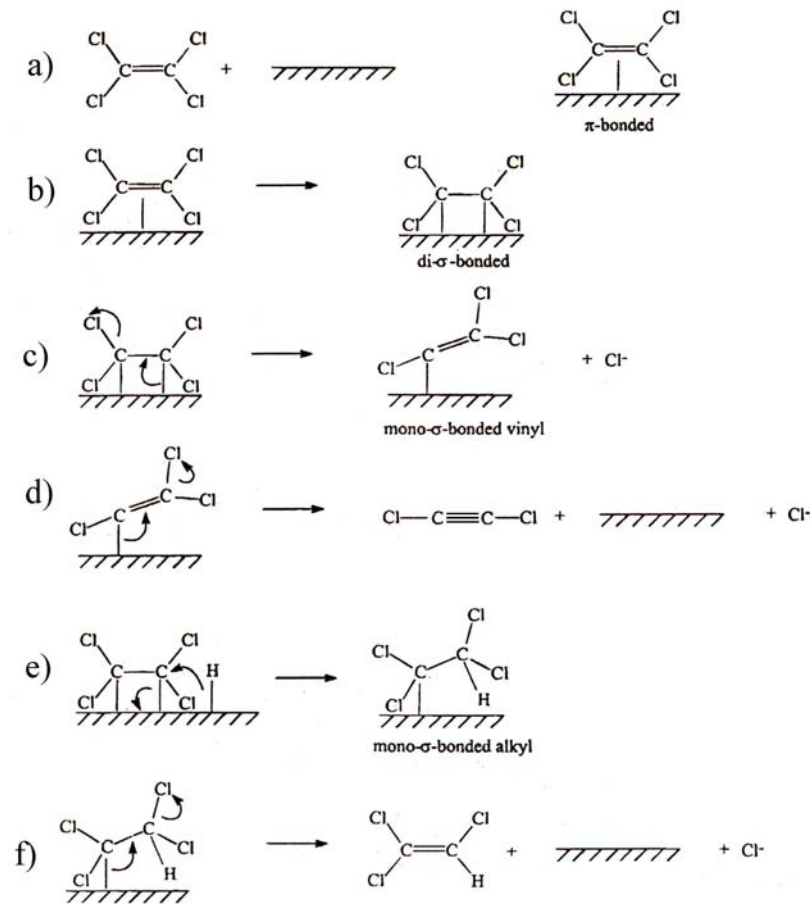
Abb. 2.1 Von ARNOLDS & ROBERTS [2000] vorgeschlagener Mechanismus für die reduktive Dechlorierung von PCE mit elementarem Eisen
