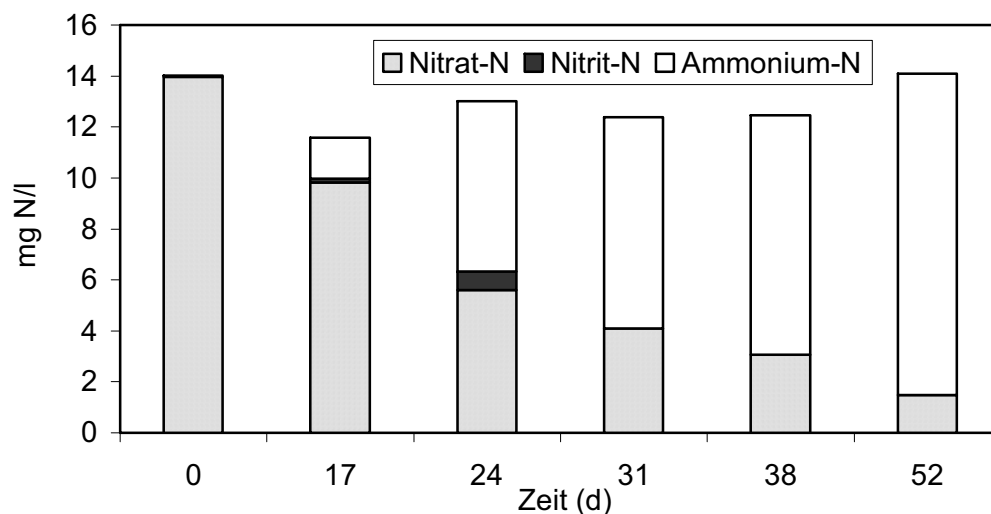
Abb. 4.3 Verlauf der Nitrat-Reduktion bezogen auf Stickstoff in abiotischen Ansätzen mit 2 Gew.-% GG.
