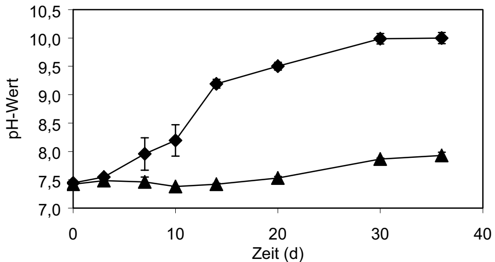
Abb. 4.13 Entwicklung der pH-Werte in carbonatgepufferten Ansätzen mit 2 Gew.-% GG (▲) und ca. 4 Gew.-% Eisenschwamm (◆).
